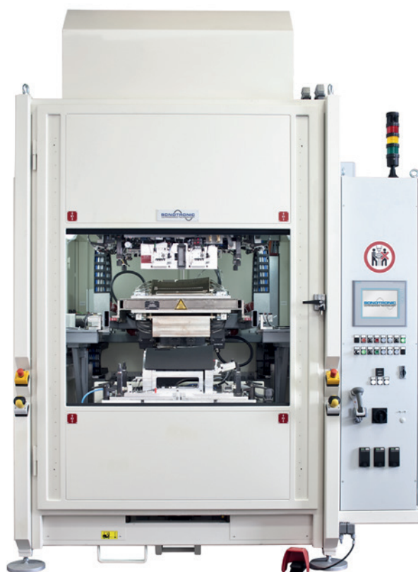
Las máquinas de elementos calefactores con eje NC horizontal o vertical son adecuadas para soldar uniones de gran superficie o carcasas dobles en piezas de trabajo hechas de termoplásticos.
